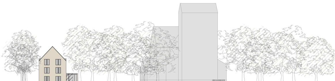
ANSICHT WESTEN M 1 : 200
