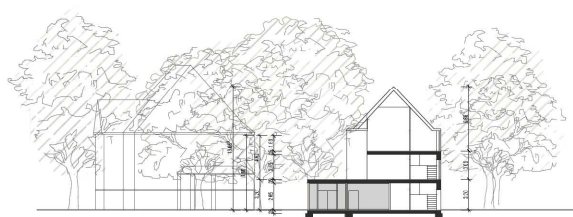
SCHNITT M 1 : 200
